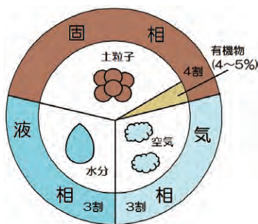
理想的な土の3相
